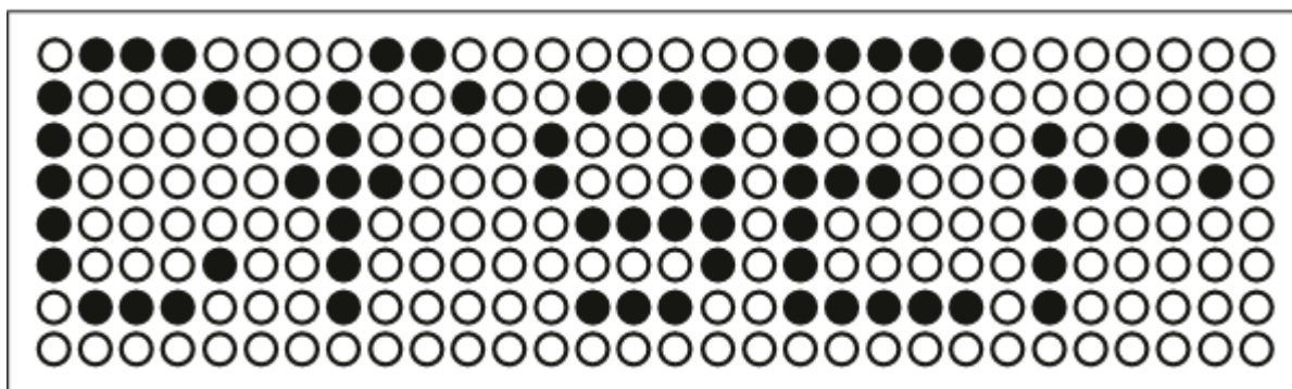
Rys. 5 Błąd konfiguracji
