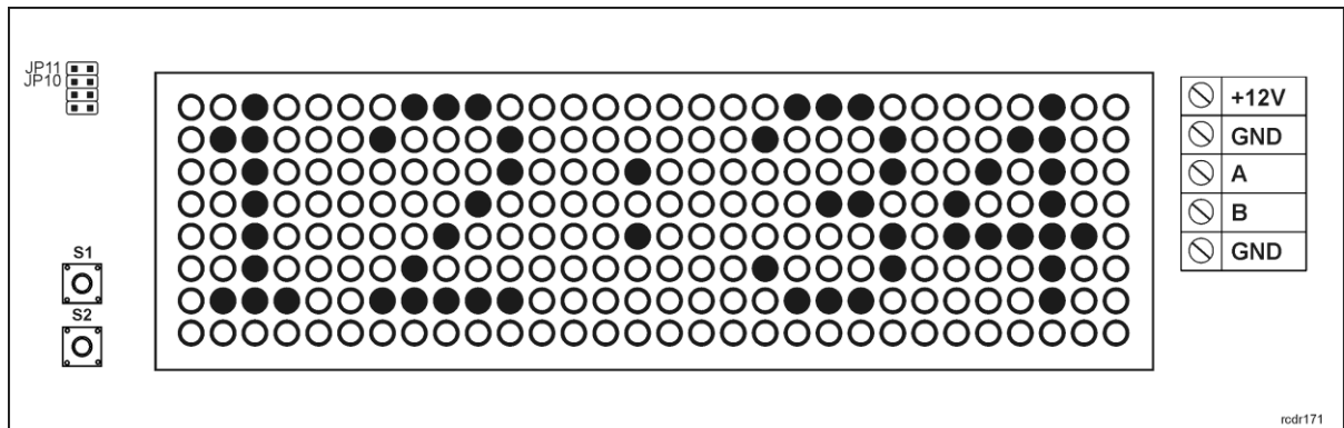
Rys. 1 Wyświetlacz ASCD-1
