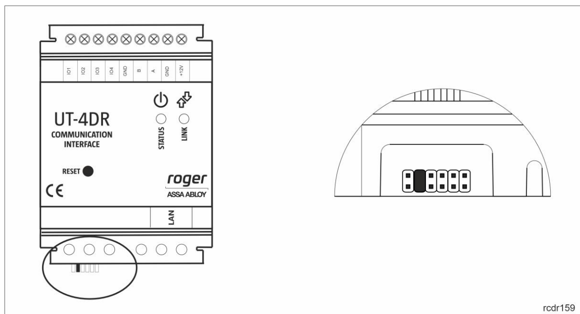
Rys.8 Lokalizacja styku zworki do resetu ustawień
