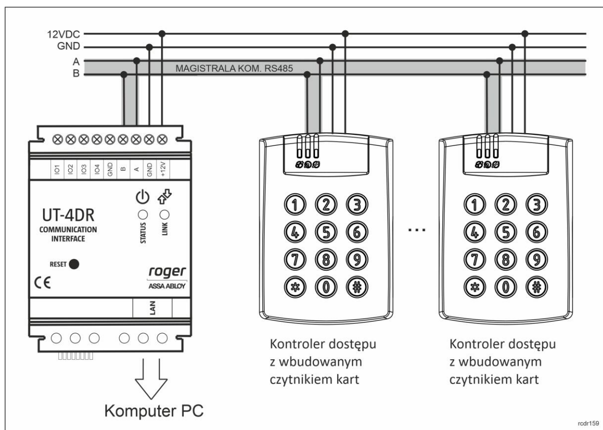
Rys. 1 Schemat typowego podłączenia interfejsu komunikacyjnego UT-4DR
