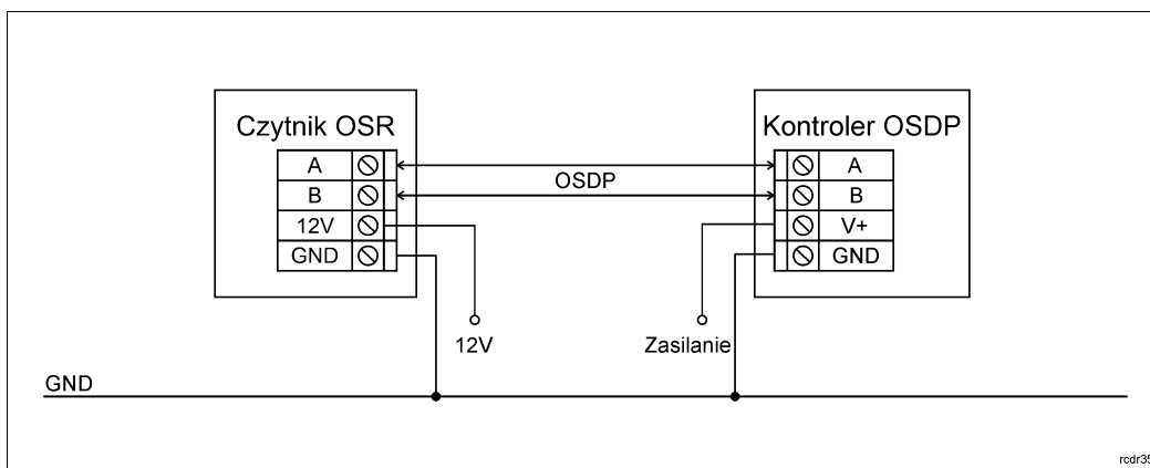
Rys. 8 Podłączenie czytnika OSR bezpośrednio do kontrolera OSDP
