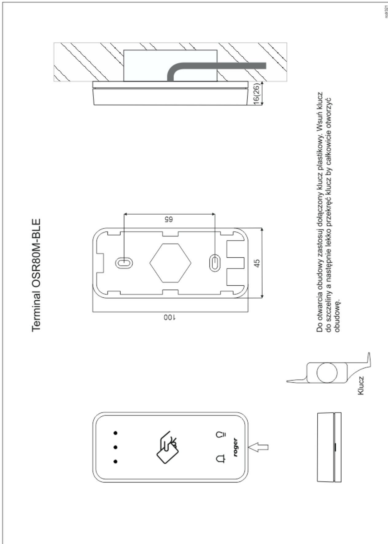
Rys. 6 Instalacja OSR80M-BLE
