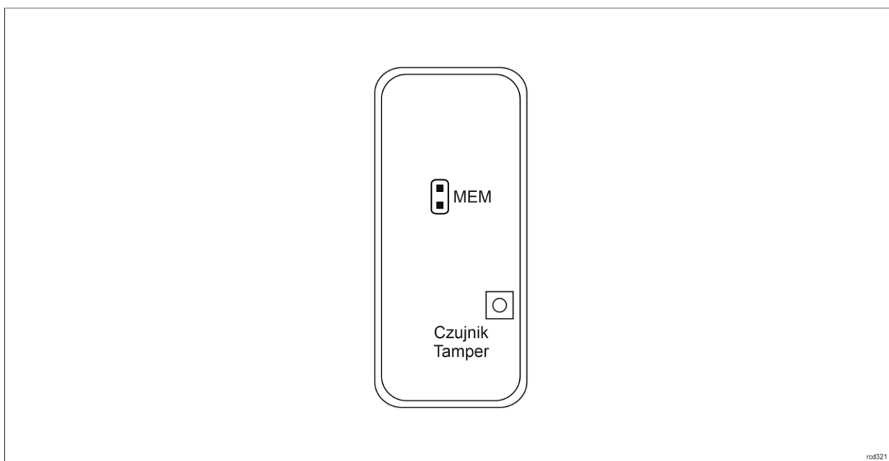
Rys. 5 Zworka programowa
