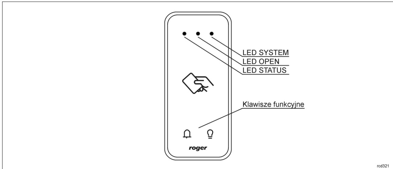
Rys. 3 Wskaźniki LED i klawisze funkcyjne
