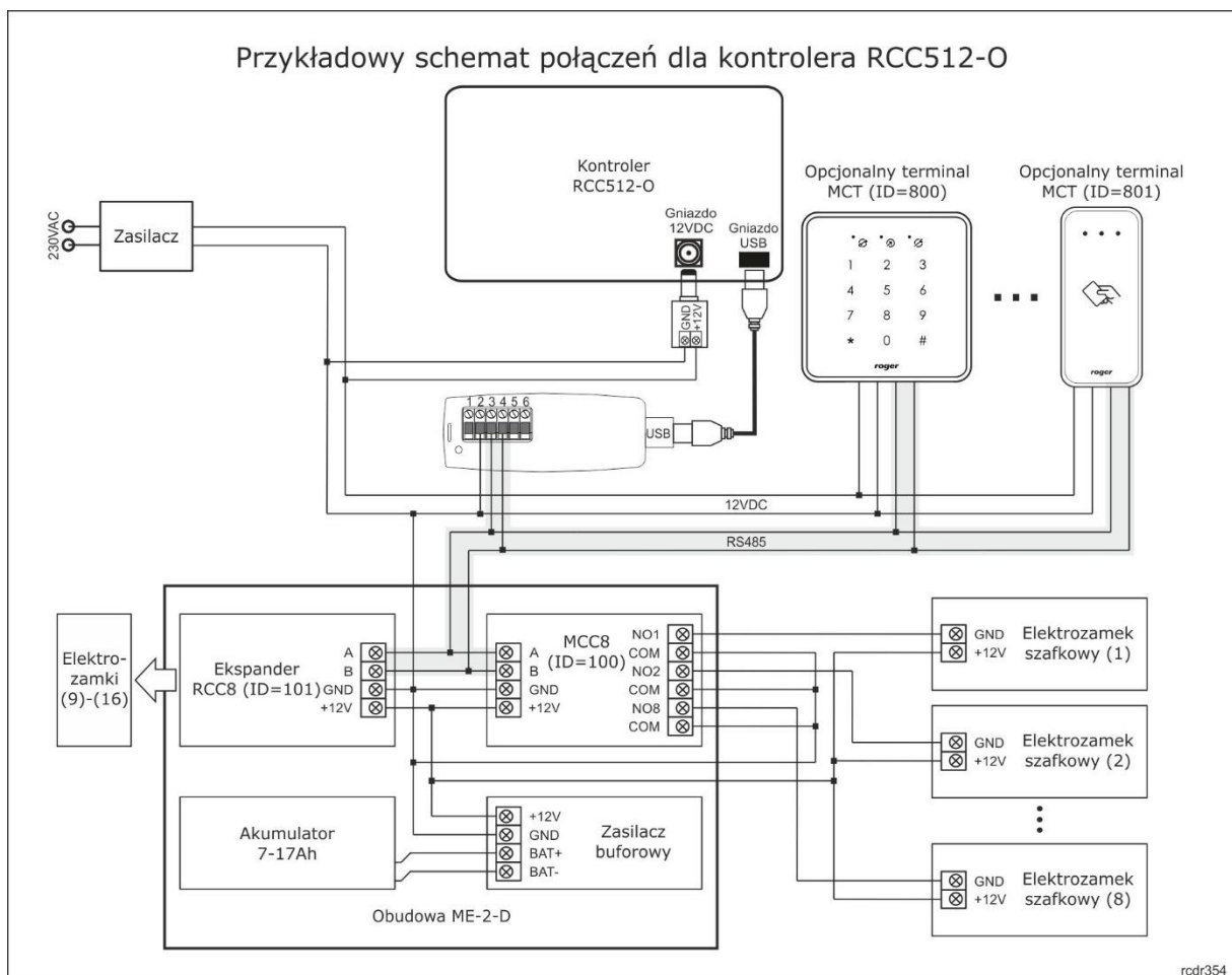
Rys. 6 Przykładowy schemat połączeń
