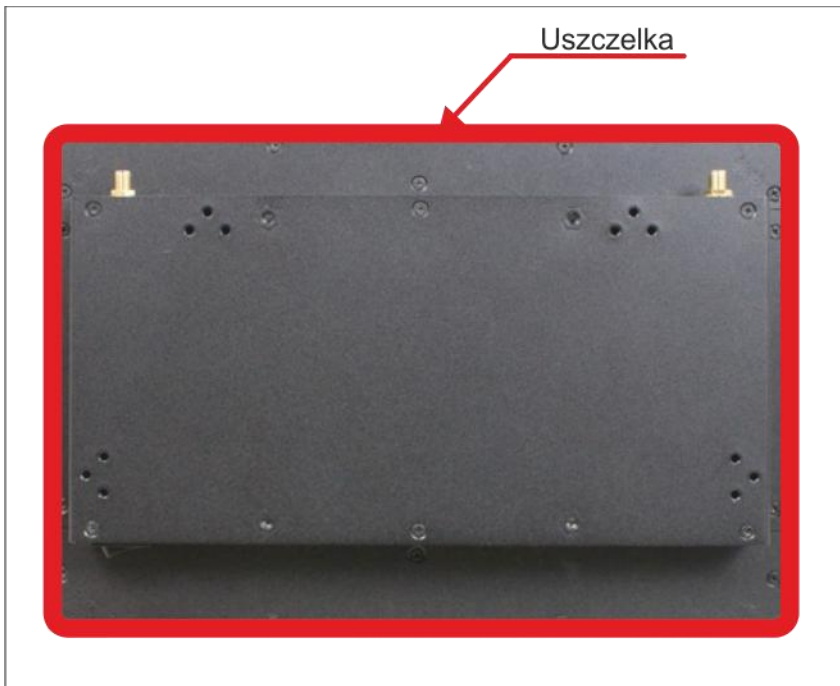
Rys. 5 Szkic ukazujący miejsce uszczelnienia przestrzeni pomiędzy kołnierzem obudowy panelu a podłożem
