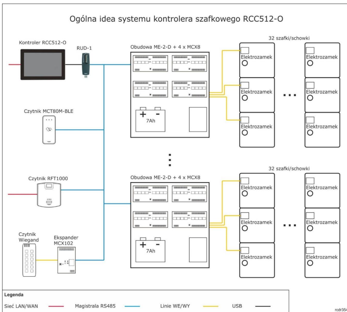
Rys. 1 Ogólna idea systemu z kontrolerem RCC512-O
