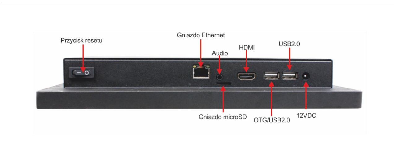
Rys. 3 Widok wejść, wyjść kontrolera RCC512-O
