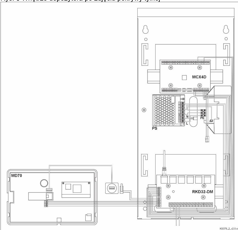
Rys. 7 Podstawa obudowy panelu kontrolnego
