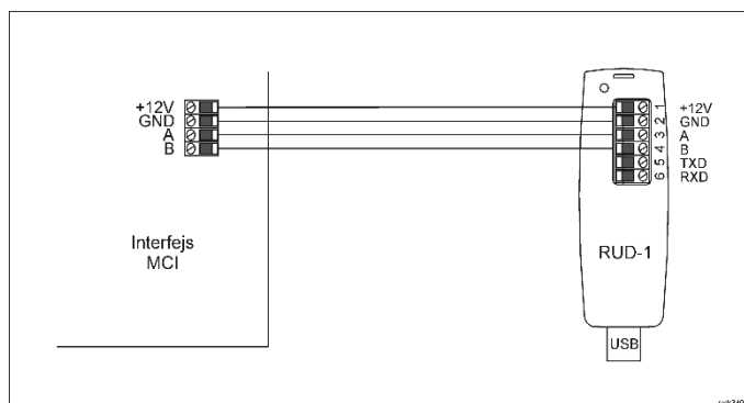
Rys. 1 Podłączenie interfejsu MCI-2 do RUD-1 w celu konfiguracji
