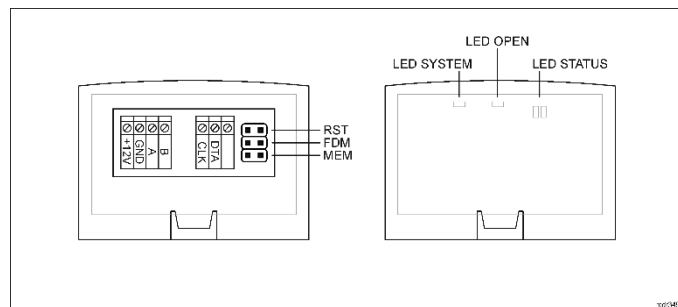
Rys. 3 Lokalizacja styków serwisowych i wskaźników LED
