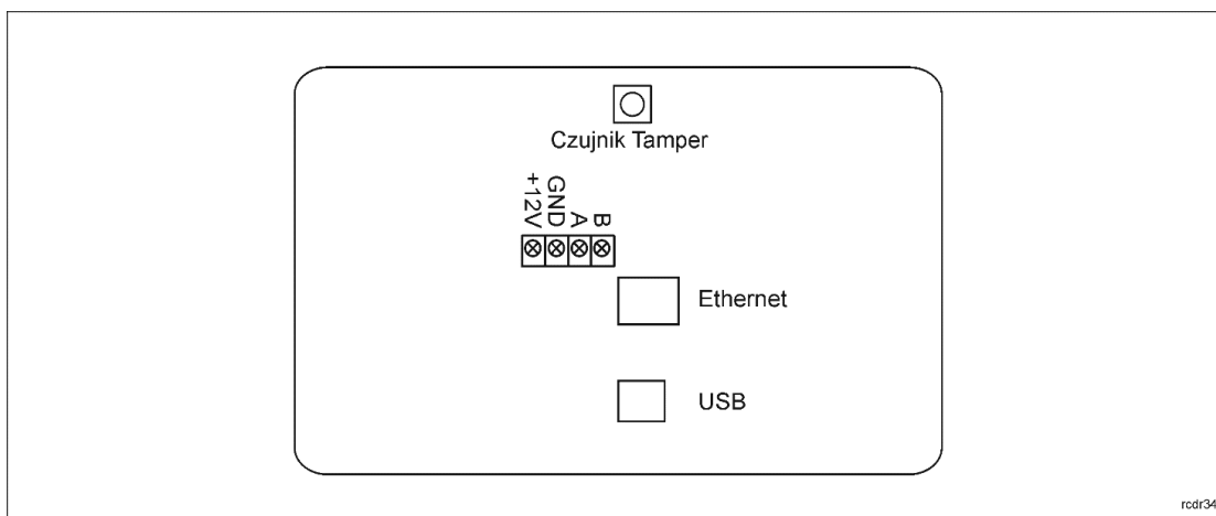
Rys. 3 Wewnętrzna strona panelu przedniego RCC512
