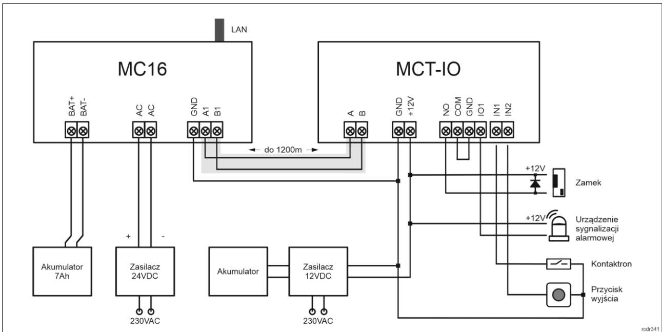
Rys. 8 Schemat przykładowego podłączenia terminala do kontrolera MC16
