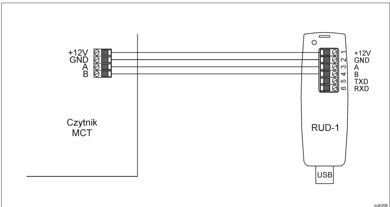
Rys. 9 Sposób podłączenia terminala do interfejsu RUD-1.
