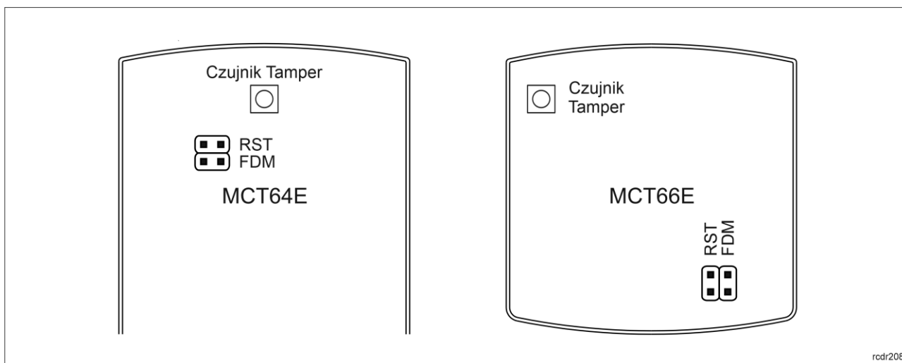
Rys. 4 Zworki programowe
