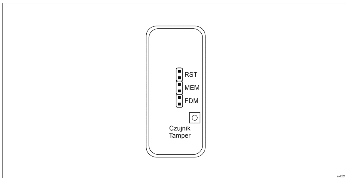
Rys. 4 Zworki konfiguracyjne
