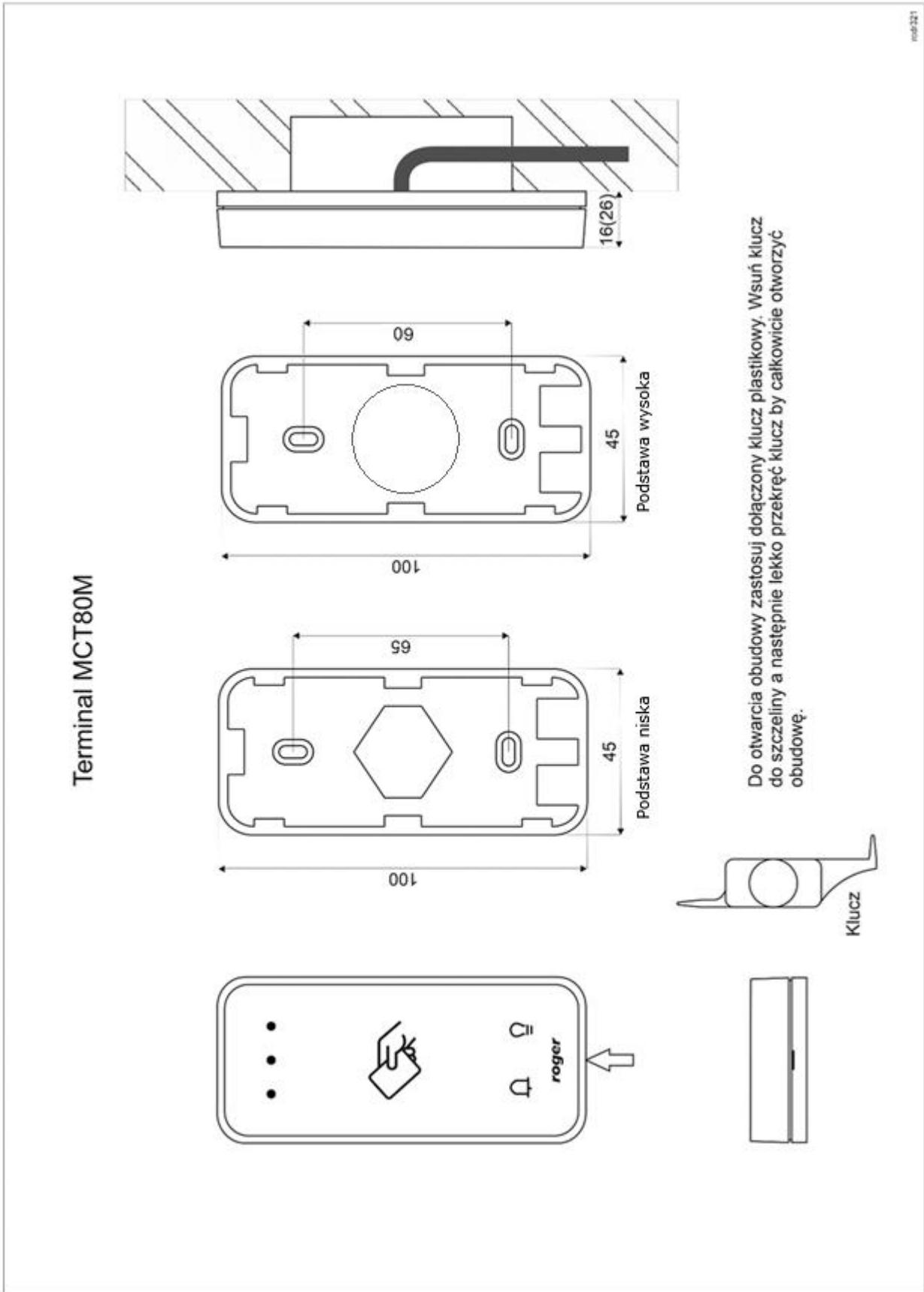
Rys. 5 Instalacja MCT80M
