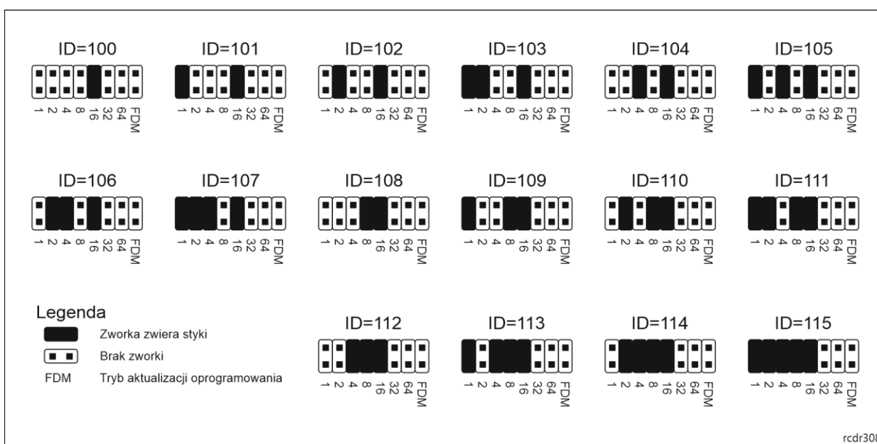
Rys. 8 Manualne ustawienie adresu ekspandera
