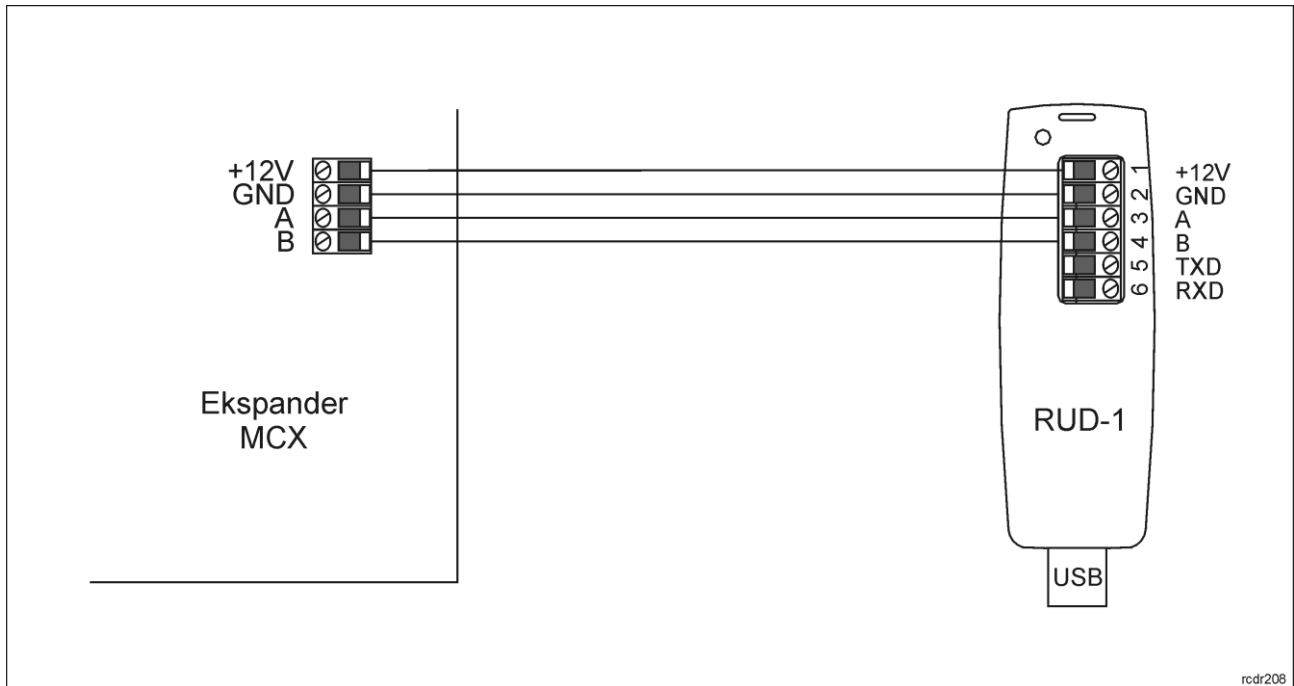
Rys. 7 Sposób podłączenia ekspandera do interfejsu RUD-1
