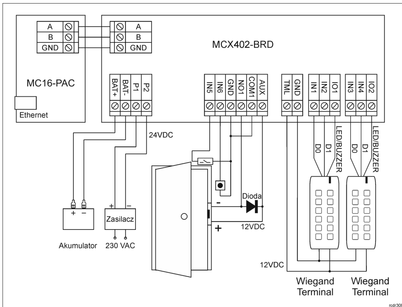
Rys. 5 Typowa obsługa przejścia z czytnikami Wiegand
