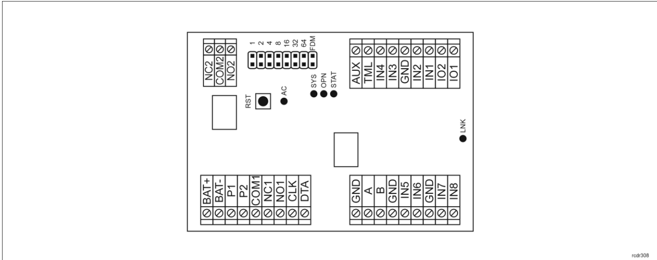
Rys. 2 Ekspander MCX402-BRD
