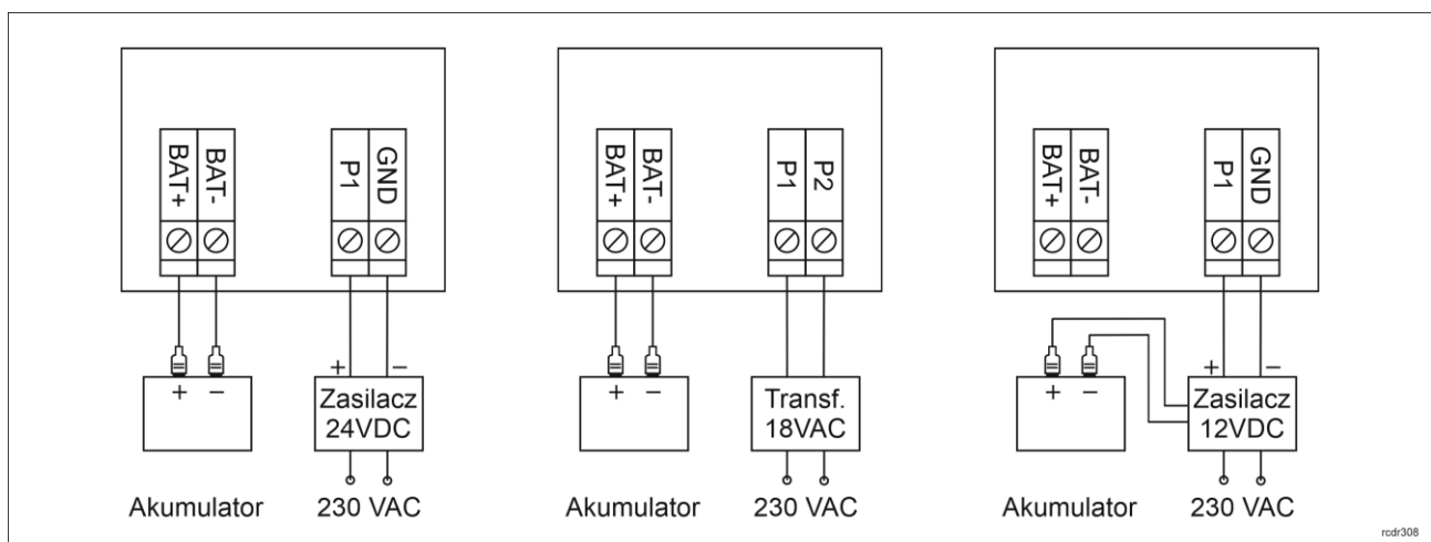
Rys. 1 Zasilanie ekspandera MCX402-BRD
