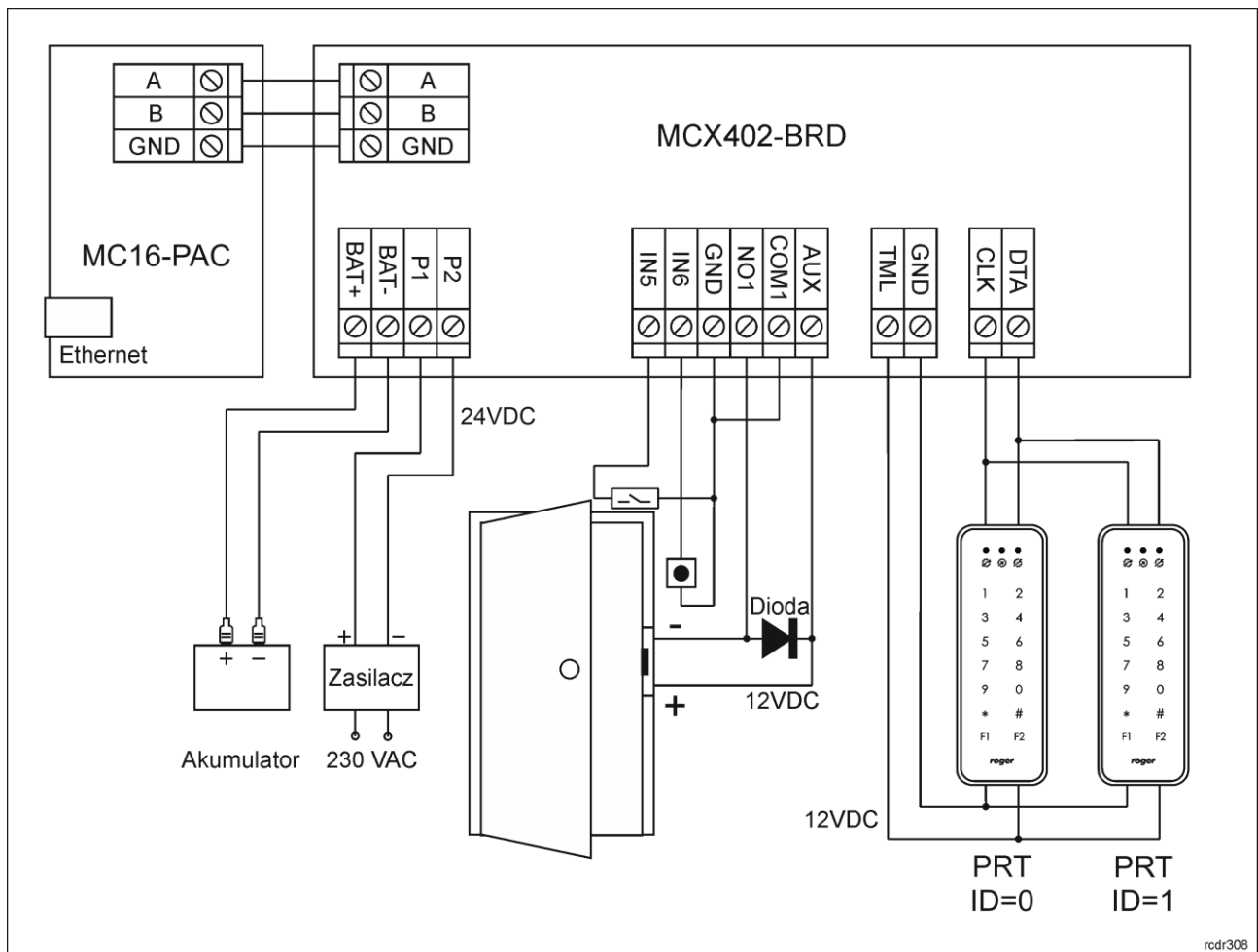
Rys. 6 Typowa obsługa przejścia z czytnikami PRT
