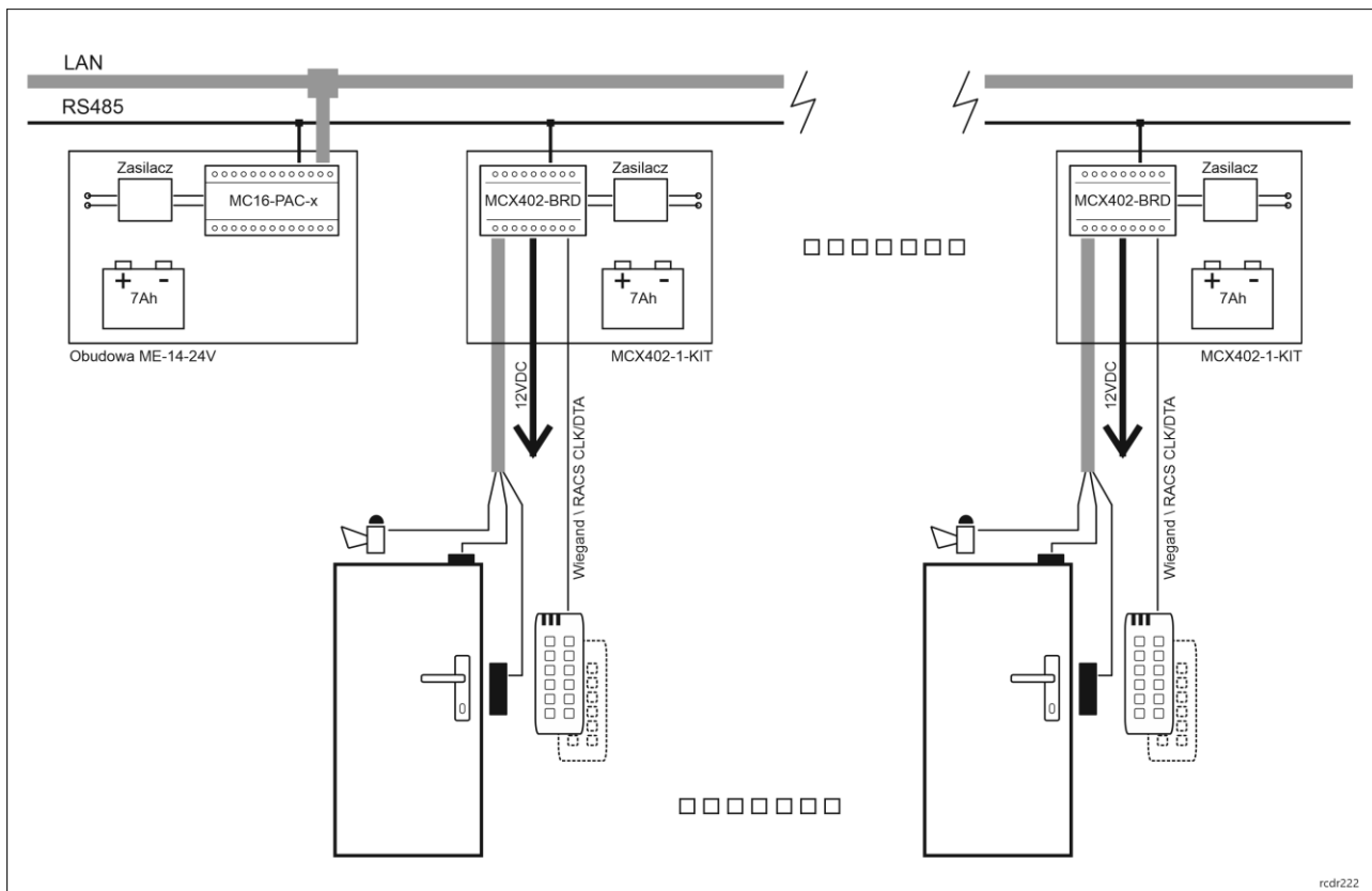
Rys. 4 Scenariusz pracy z zestawami MCX402-1-KIT
