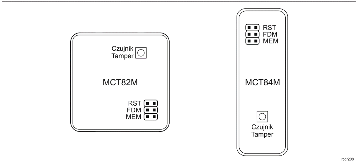
Rys. 4 Zworki konfiguracyjne
