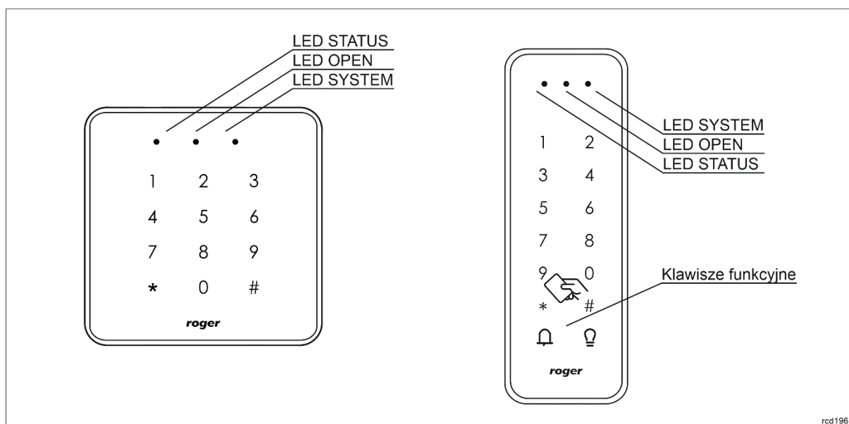
Rys. 3 Wskaźniki LED
