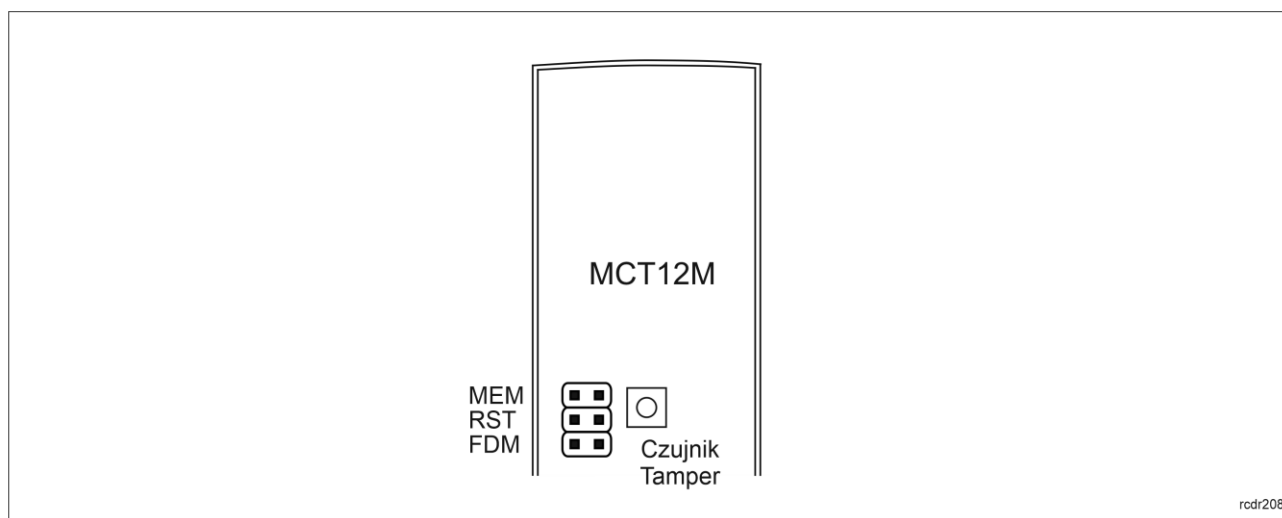
Rys. 3 Zworki programowe
