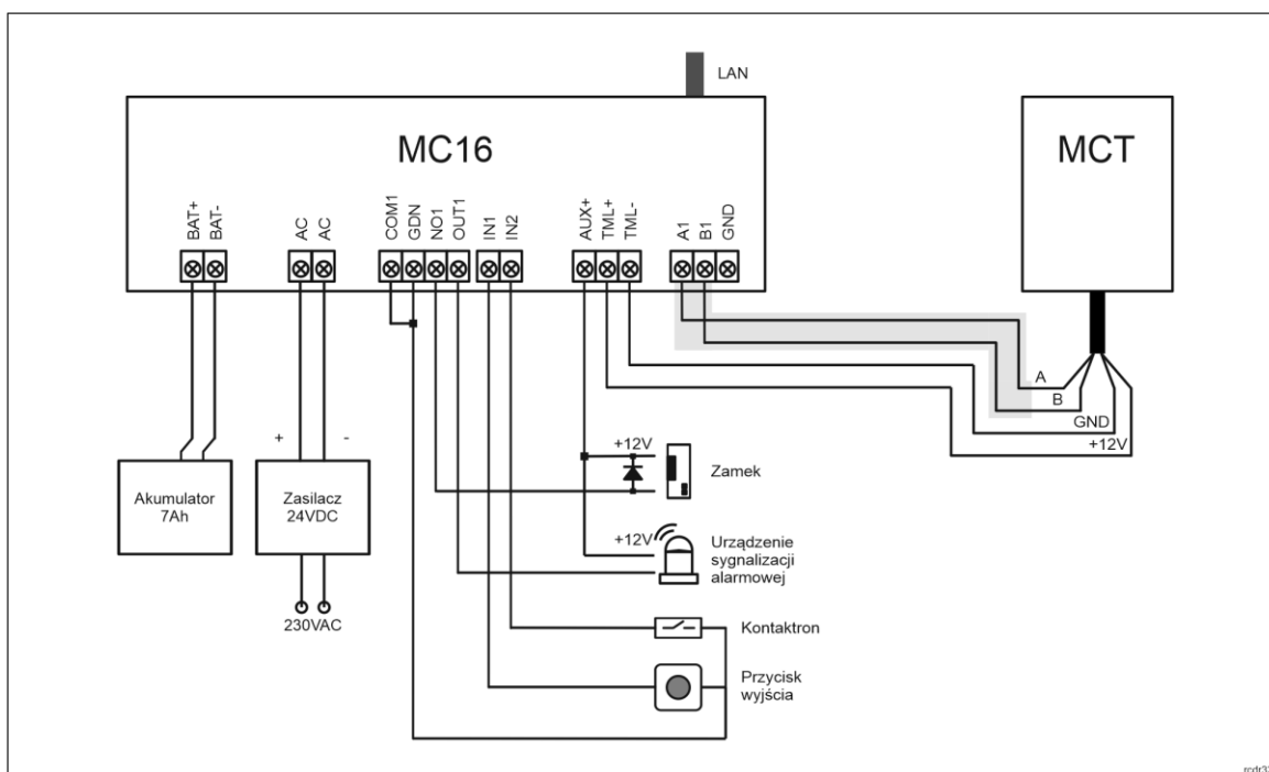
Rys. 5 Schemat przykładowego podłączenia terminala do kontrolera MC16
