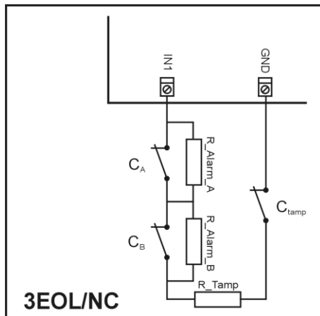
Rys. 12 Wejście typu 3EOL/NC
