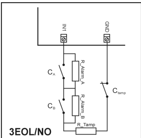
Rys.11 Wejście typu 3EOL/NO
