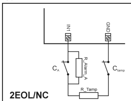
Rys. 10 Wejście typu 2EOL/NC
