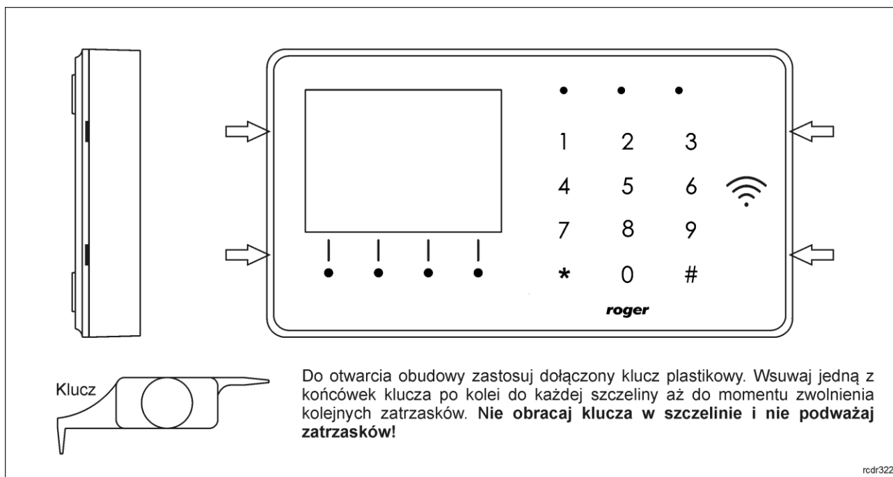
Rys. 14 Demontaż obudowy urządzenia
