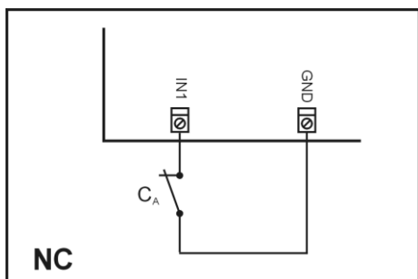
Rys. 6 Wejście typu NC
