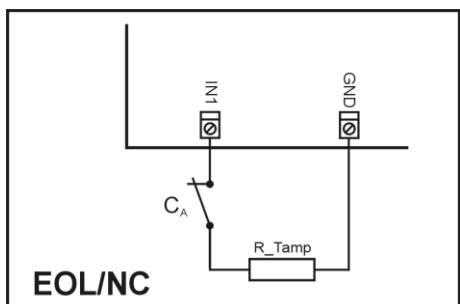
Rys. 8 Wejście typu EOL/NC
