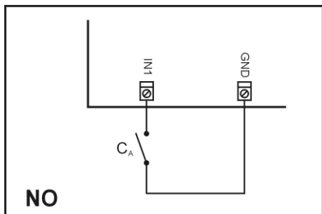
Rys. 5 Wejście typu NO
