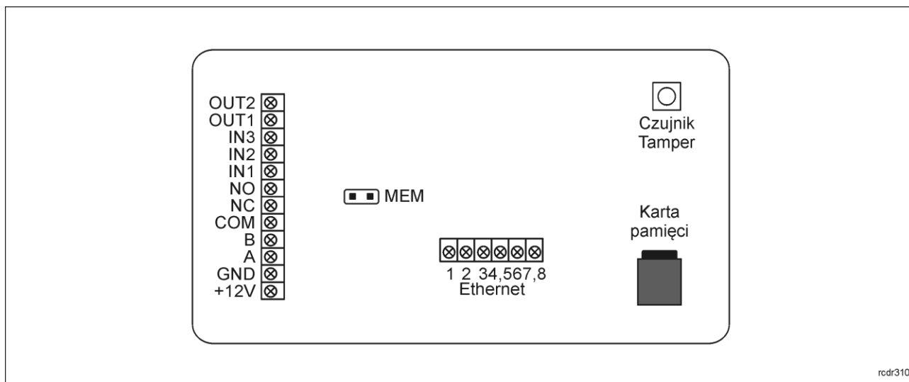
Rys. 15 Wewnętrzna strona panelu przedniego
