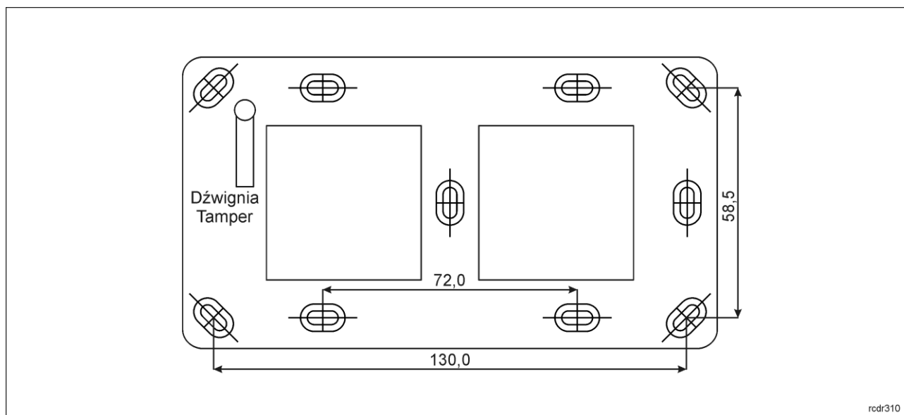
Rys. 16 Panel tylny
