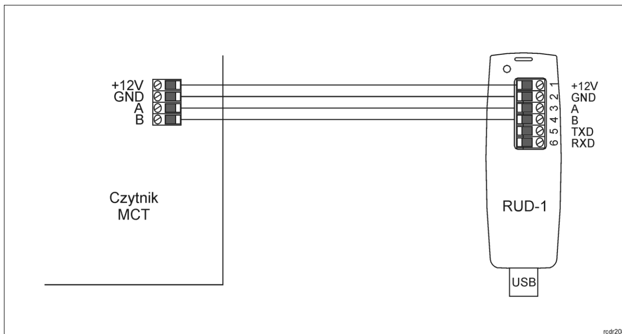
Rys. 17 Sposób podłączenia terminala do interfejsu RUD-1.
