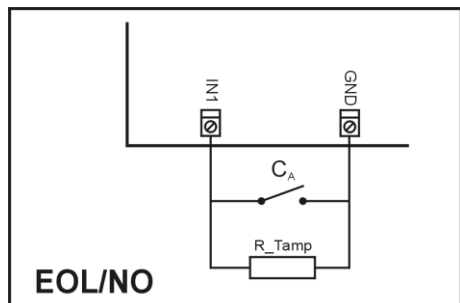
Rys. 7 Wejście typu EOL/NO
