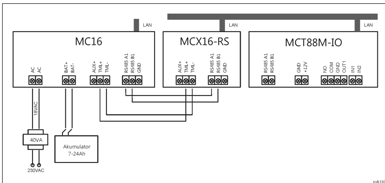
Rys. 3 Podłączenie terminala do kontrolera MC16 poprzez interfejs MCX16-RS
