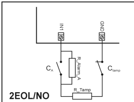
Rys. 9 Wejście typu 2EOL/NO
