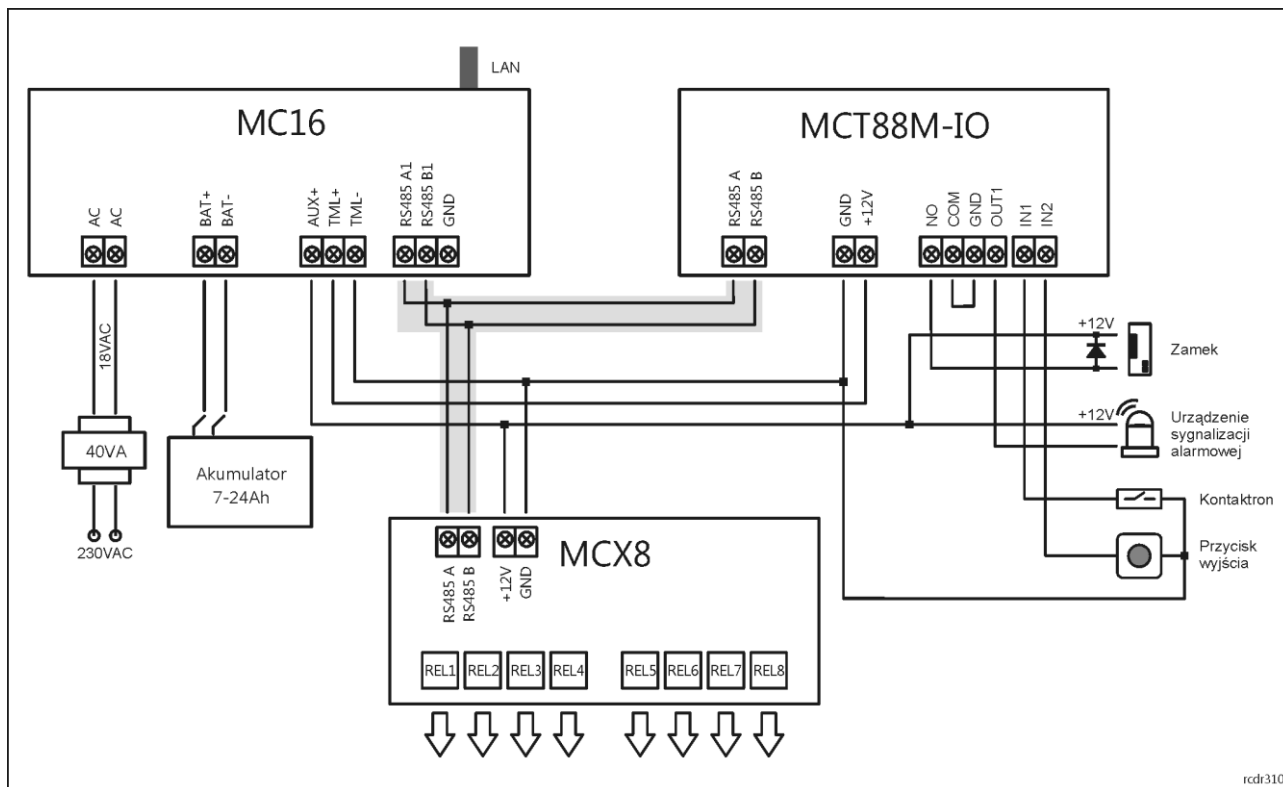
Rys. 17 Schemat przykładowego podłączenia terminala do kontrolera MC16
