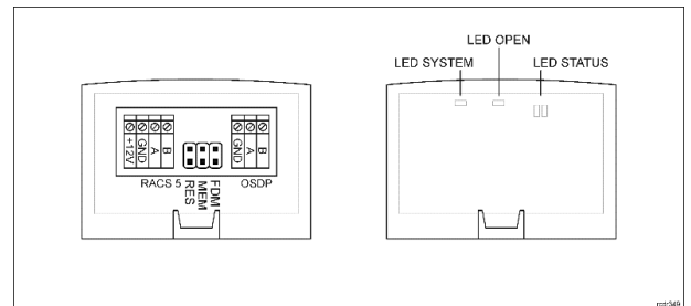
Fig. 3 MCI-3 interface
