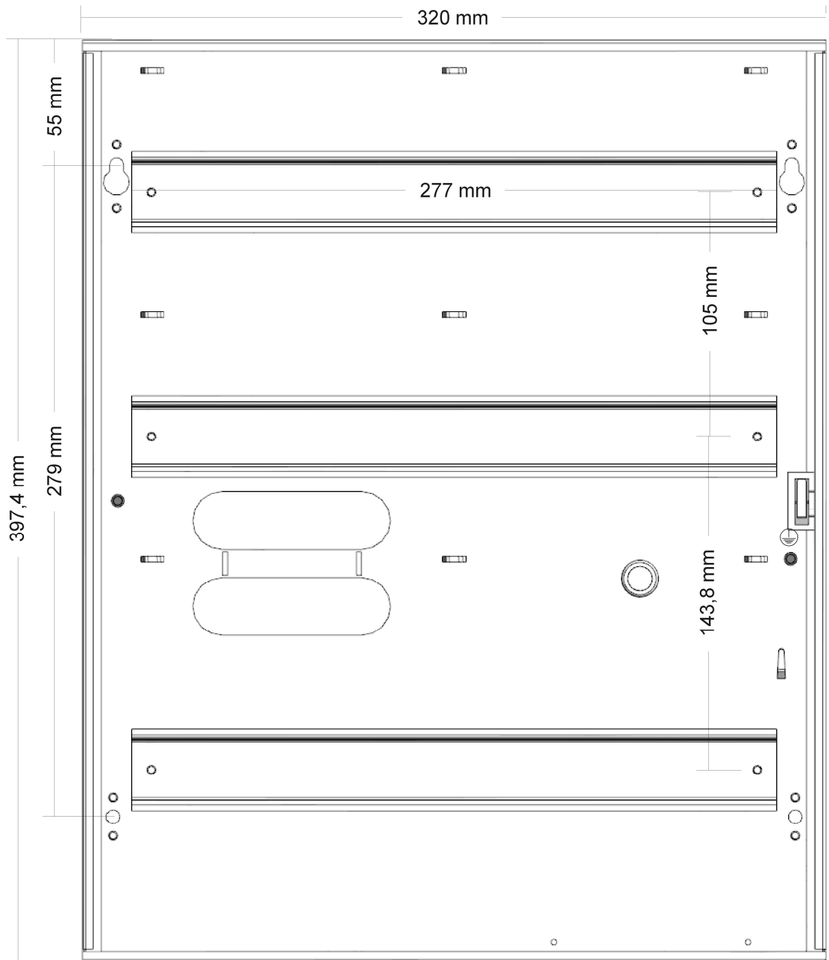
Fig. 4 ME-2-D dimensions
